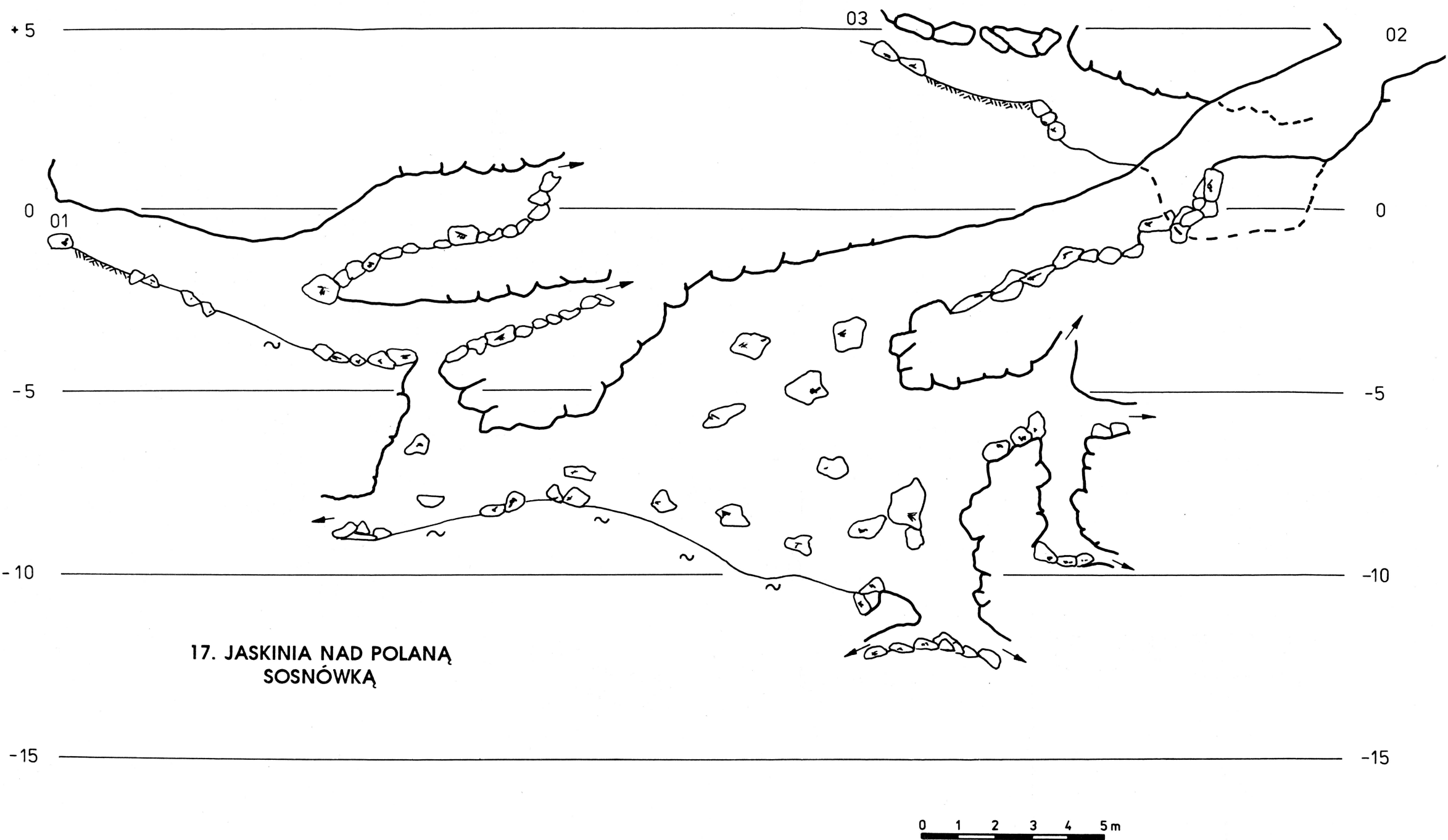
Ryc. 29. Jaskinia Nad Polaną Sosnówką – przekrój rozwinięty (pomiary: A. Amirowicz, M. Gradziński, plan: A. Amirowicz). Nad Polaną Sosnówką cave – extended section (survey: A. Amirowicz, M. Gradziński, plan: A. Amirowicz).
